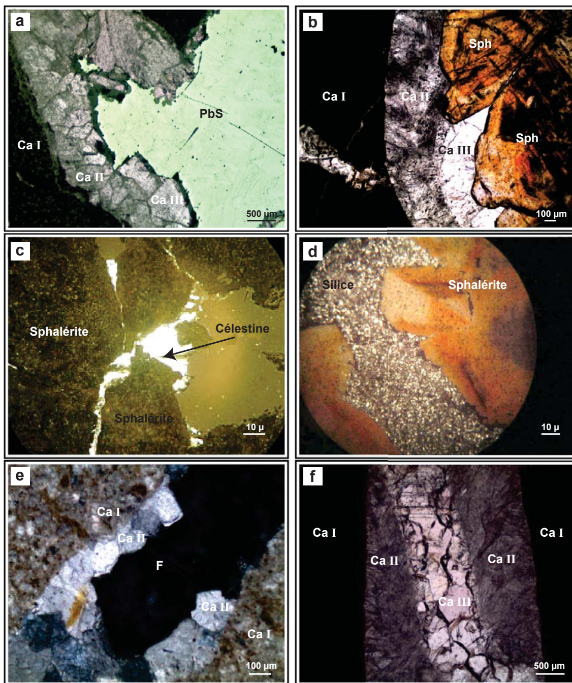
Pl. 3- Observations microscopiques de la minéralisation de l'anticlinal du Djebel Lassel : a. (LR) Plage de galène tardive avec des contours d'altération. b. (LPNA) Plage de sphalérite tardive dans une fracture. c. (LPNA) Céléstine tardive recoupant la sphalérite. d. (LPA) Poches de dissolutions à remplissage de petits grains de quartz montrant une silicification tardive. e. (LPA) Cristaux de fluorite tardive dans une fracture. f. (LPA) Différentes générations de calcite, diagenétique (CaI) et fissurale (CaII et CaIII). (LR) : lumière réfléchiée polarisée.
