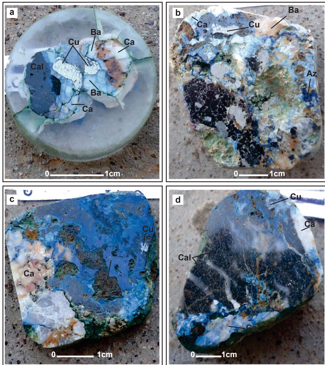
Fig. 7- Sections polies de fragment de brèches montrant l'emplacement de la minéralisation (barytine et cuivre gris).
