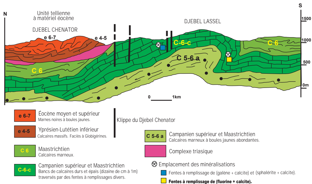
Fig. 5- Coupe géologique de l'anticlinal du Djebel Lassel avec la klippe du Djebel Chenator. Coupe extraite de la carte géologique de Kherrata n°70 (Sonatrach, 1977; modifiée).
