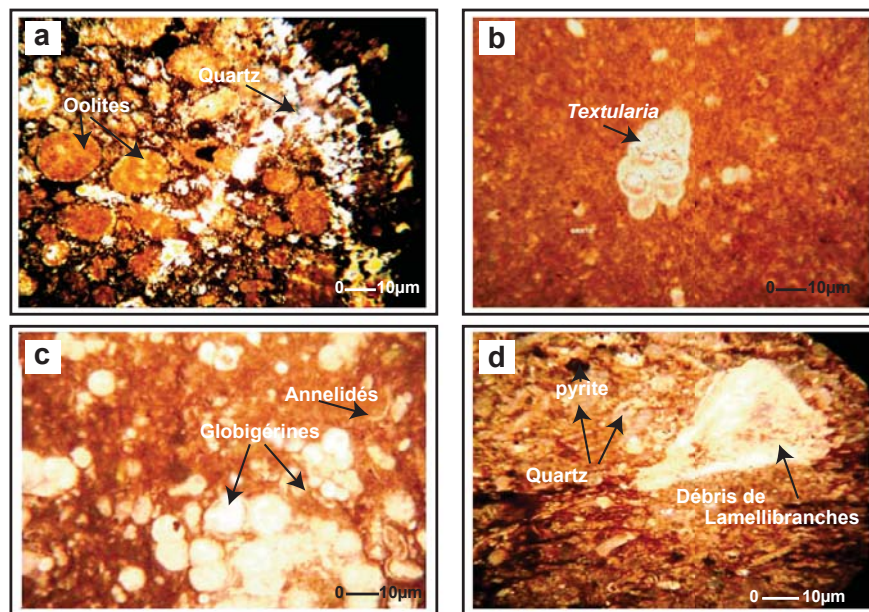
Pl. 1- Aspect microscopique des calcaires de la nappe de Djemila. a. (LPA) (LM Dj10) : calcaire oolithique du Djebel Amar Rhedou à Djermouna. b. (LPA) (LM SY1) : calcaire micritique à sections de Textularia , de Globigérines et d'Annélides. c. (LPNA) (LM SY2). d. (LPA) (LM LC13) : calcaire micritique du Djebel Lassel à débris de Lamellibranches et à cristaux de quartz abondants.
