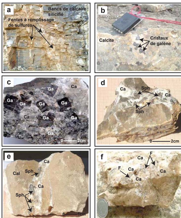
Fig. 10- Aspects macroscopiques de la minéralisation sulfurée et de la minéralisation fluorée dans les fentes de l'anticlinal du Dejbhel Lassel. a. Faciès carbonaté constitué de bancs métriques de calcaire silicifié recoupés par des fentes à remplissage divers. b et c. Cristaux automorphes de galène associée à la calcite tapissant les parois des fentes de tensions. d et e. Fractures à remplissage de calcite et de cristaux globuleux de sphalérite. f. Fente traversée par de la calcite et des petits cristaux tardifs de fluorite. ( Ga : galène; Ca : calcite; Sph : sphalérite; Cal : calcaire; F : fluorite).
