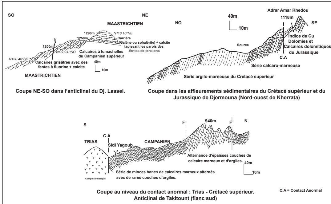
Fig. 2- Coupes dans les formations de la nappe de Djemila (région de Kherrata) (Mazari, 2005). Les datations données ont été établies par les géologues de l'ORGM (2002).
