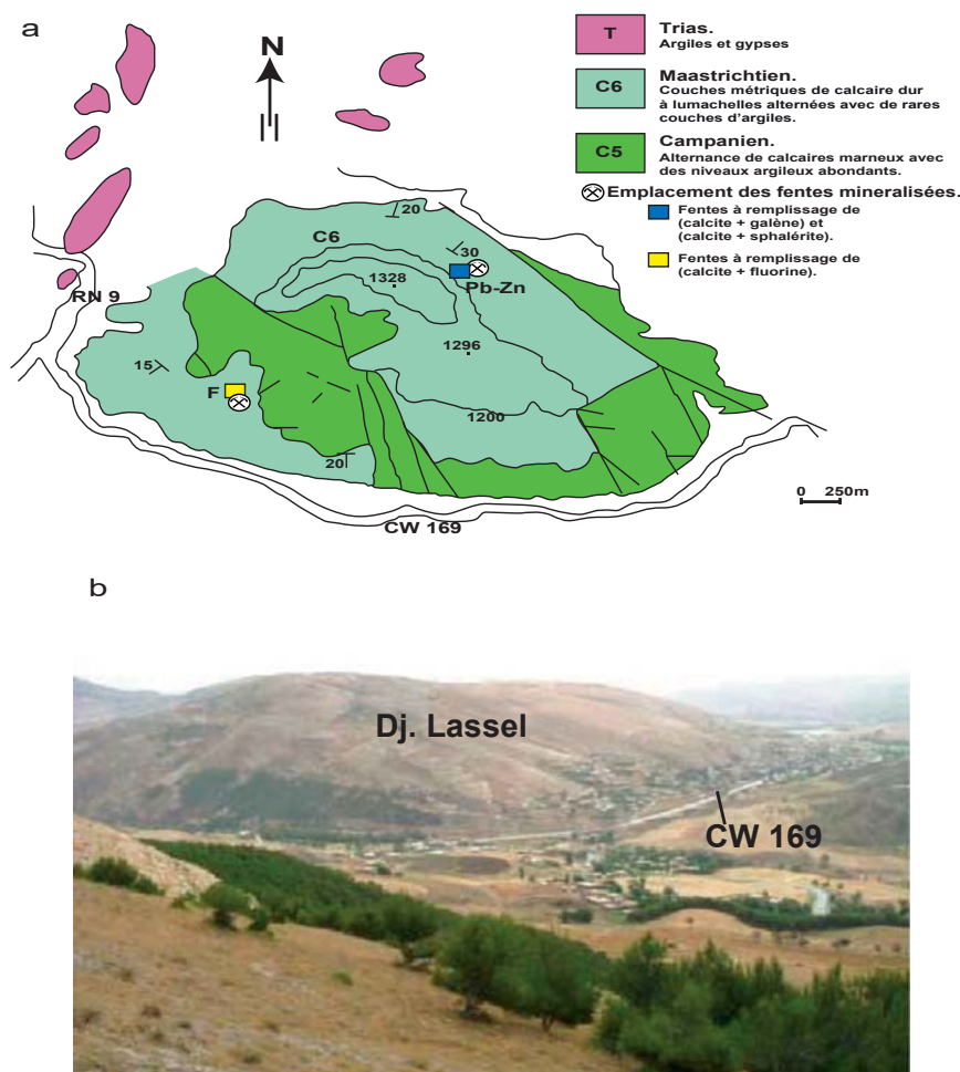
Fig. 9- a. Schéma géologique de l'anticlinal du Djebel Lassel et localisation des fentes minéralisées, établi d'après la carte géologique de la feuille de Kherrata au 1/50 000. (ORGM, 2002; modifiée).
