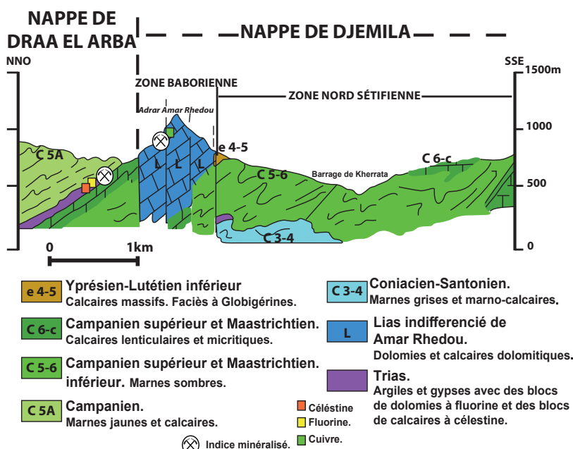
Fig. 4A- Coupe géologique dans la zone de Djermouna. Coupe extraite de la carte géologique de Kherrata n°70. (Sonatrach, 1977; modifiée).
