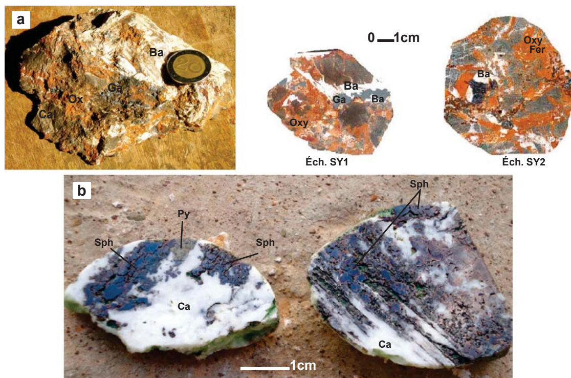
Fig. 8- Aspect macroscopique de la minéralisation dans l'anticlinal de Takitount. a. Brèche tectonique constituée de fragments de calcaire noir (cal) à galène (Ga), barytine (Ba) et oxydes de fer (Oxy). Les cristaux de galène apparaissent automorphes (Échs. SY1 –SY2) et sont associés à la barytine précoce. b. Échantillons de profondeur, à 66 m (Éch. SO6 (66) montrant des plages de sphalérite (Sph), de calcite (Ca) et de petits cristaux de pyrite (Py) occupant le ciment de la brèche).
