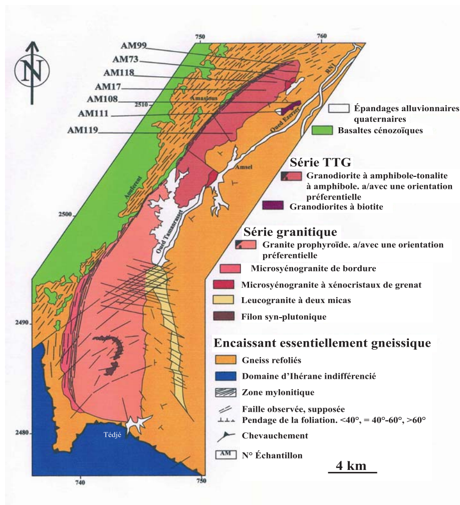
Fig. 2 - Carte géologique du batholite composite de l'Amsel (modifiée d'après Bouzeguella-Talmat et Ouabadi, 2002) Geological map of the Amsel composite batholiths (modified from Bouzeguella-Talmat and Ouabadi, 2002)
