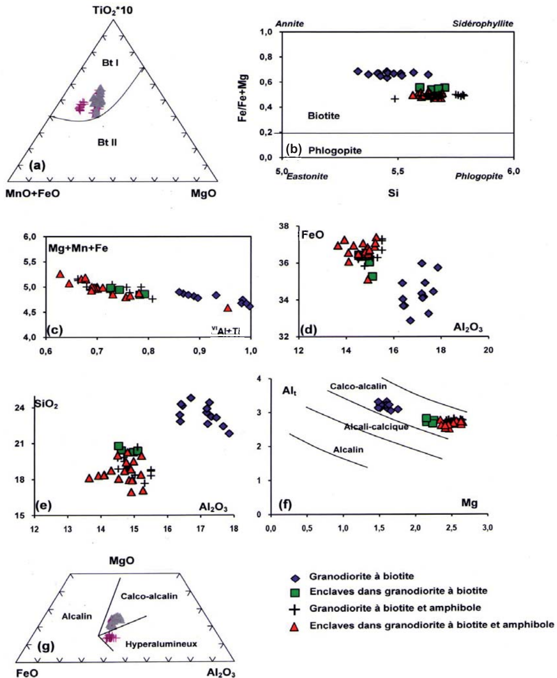
Fig. 7 - (a) Biotite des granodiorites hôtes (croix) et des enclaves (losange) dans le diagramme de Nachit et al. 1985 ( Biotite in granodiorite (cross) and their enclaves (lozenge) plotted in the Nachit and al. (1985) diagram ). (b) Composition des biotites des granodiorites et des enclaves dans le diagramme de Deer et al. 1980 ( Biotite in granodiorite and their enclaves plotted in the Deer et al. (1980) diagram ). (c) Substitution dans le site octaédrique des biotites ( Substitution in biotite octahedral site ). (d,e) Diagrammes SiO_2/Al_2O_3 , FeO/Al_2O_3 des biotites ( Bivariate plots of the oxides SiO_2 , FeO , vs Al_2O_3 ). (f) Compositions des biotites dans le diagramme de Nachit et al. 1985 ( Biotite compositions in the Nachit and al. (1985) diagram ). (g) Compositions des biotites dans le diagramme ternaire Al_2O_3 - FeO - MgO de Abdel-Rahman (1994) ( Biotite compositions in the Abdel-Rahman (1994) Al_2O_3 - FeO - MgO ternary diagram ).
