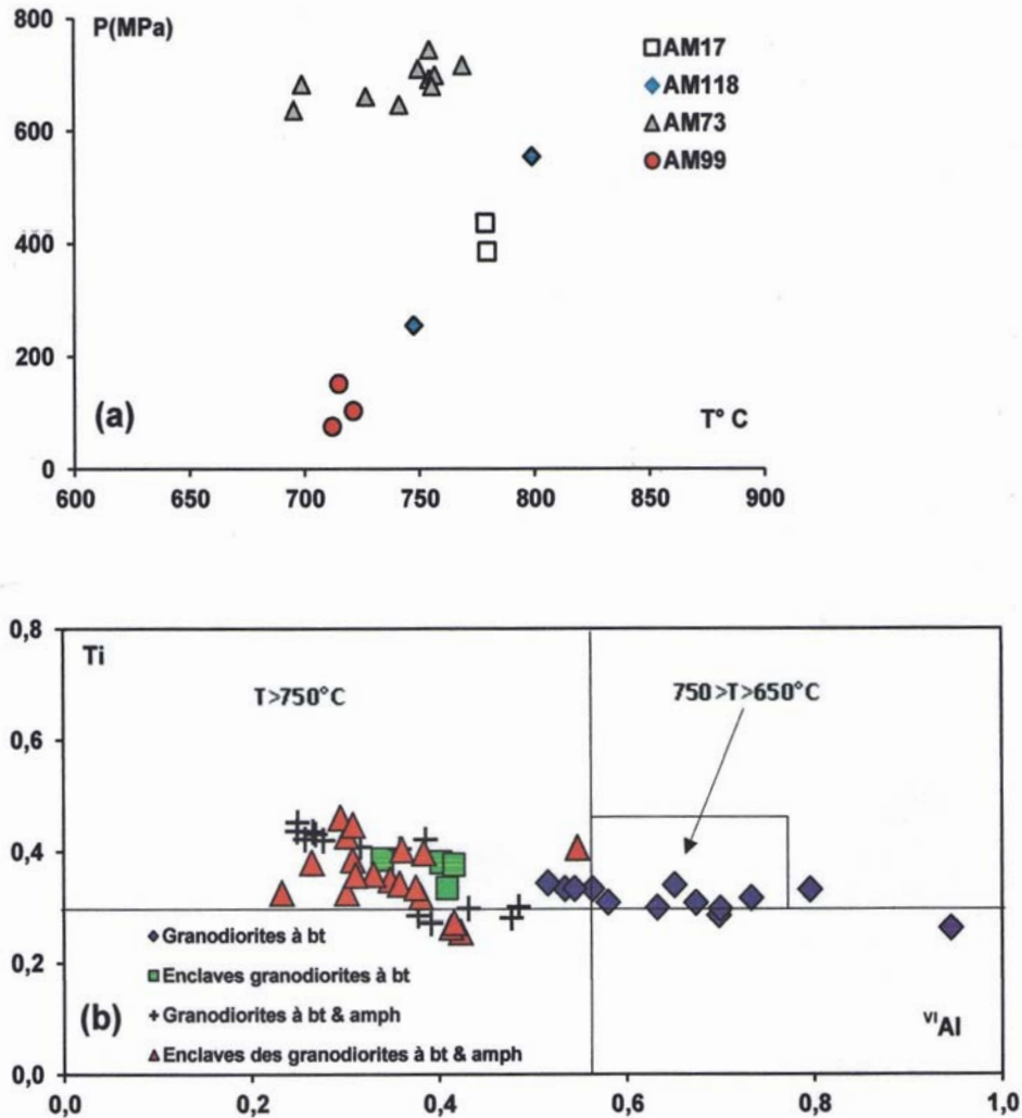
Fig. 8 - (a) Diagramme P-T dans les amphiboles ( P-T diagram in amphibole ). (b) Diagramme de Schreurs (1985) ( Schreurs diagram (1985) ).
