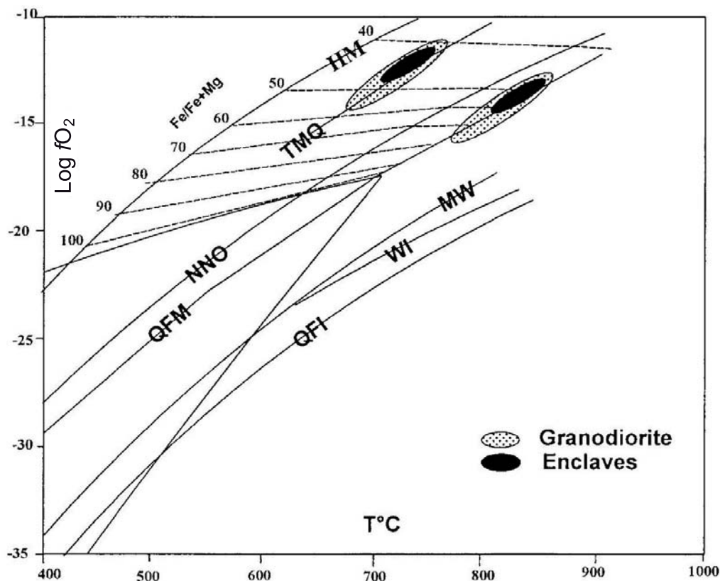
Fig. 9 - Diagramme fugacité d'oxygène - température.
