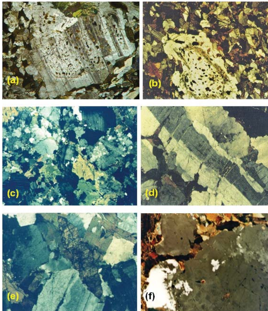
Fig. 4 - Aspect au microscope polarisant de certains minéraux caractéristiques. Thin sections photographs of typical crystals.
