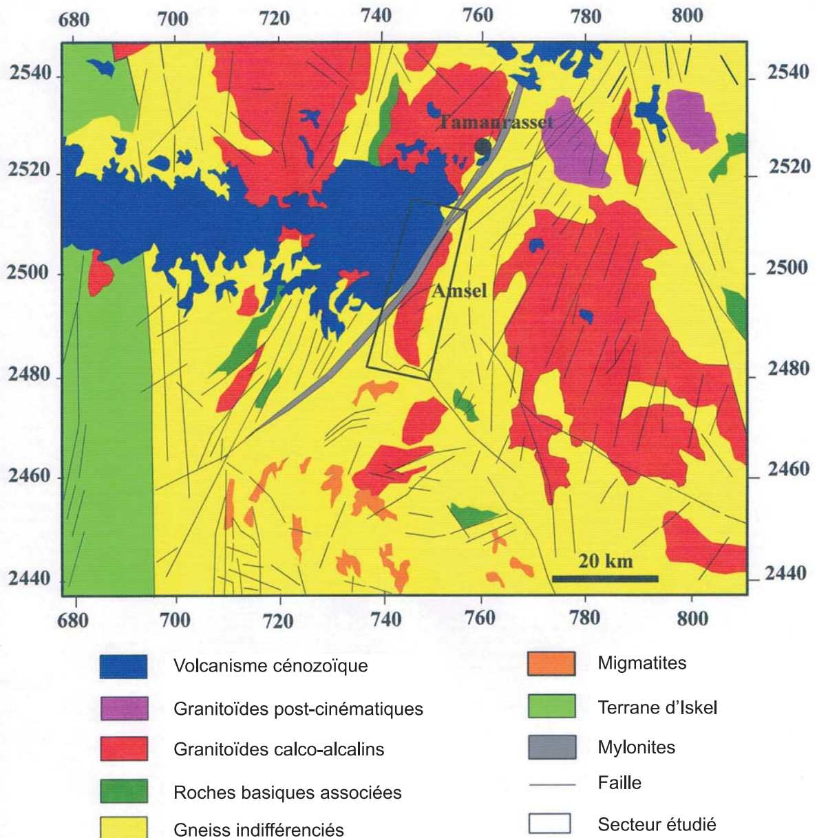
Fig.1 - Situation et cadre géologique du batholite de l'Amsel (carte au 1/200.000, feuille Tamanrasset, ORGM, 2002)
