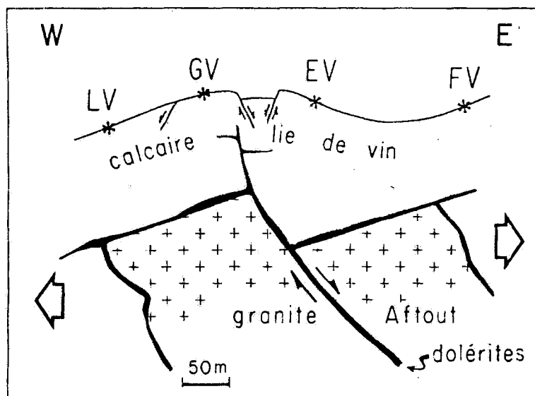
Fig. 6 - Interprétation structurale expliquant la formation du « pli » de Tilemsi.
