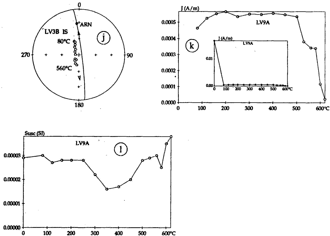
Fig. 2 - Projection à aire égale (a) des directions d'ARN des sites LV, GV, EV, FV et leur histogramme d'intensité d'ARN (b) et de susceptibilité magnétique (c) correspondantes. Cercle ouvert (fermé): projection sur l'hémisphère supérieur (inférieur). n = nombre d'échantillons. Projection orthogonale (Zijderveld, 1967) des désaimantations thermiques (d-h) d'échantillons montrant la présence de deux composantes d'aimantation: une composante visqueuse détruite avant 160°C et une composante haute température jusqu'à 560-620°C. Cercle ouvert (fermé): projection sur le plan vertical (horizontal). Pour les échantillons présentés en (d), (e), (g) et (h), l'ARN n'est représentée que sur une petite échelle car à 80°C, on a détruit plus de 80% de la rémanence (i, k). Par contre pour l'échantillon présenté en (f), on n'en a détruit que 50-60% du signal magnétique. Ceci est caractéristique de la destruction de la goéthite à moins de 200°C (voir fig. 4). Notons cependant, que la désaimantation par champs alternatifs à 0.1 T n'a pas permis d'isoler une composante d'aimantation caractéristique (g). Projection à aire égale de la désaimantation d'un échantillon le long d'un grand cercle de réaimantation (j), montrant la direction à atteindre (« stable end point ») représentée par des flèches (voir tableau II). La direction de l'ARN coïncide bien avec le champ dipôle actuel. La destruction de plus de 80% de la rémanence (k) est également accompagnée par une transformation minéralogique vers 250-400°C (l), probablement liée à la présence de sulfures de type pyrrhotite.
