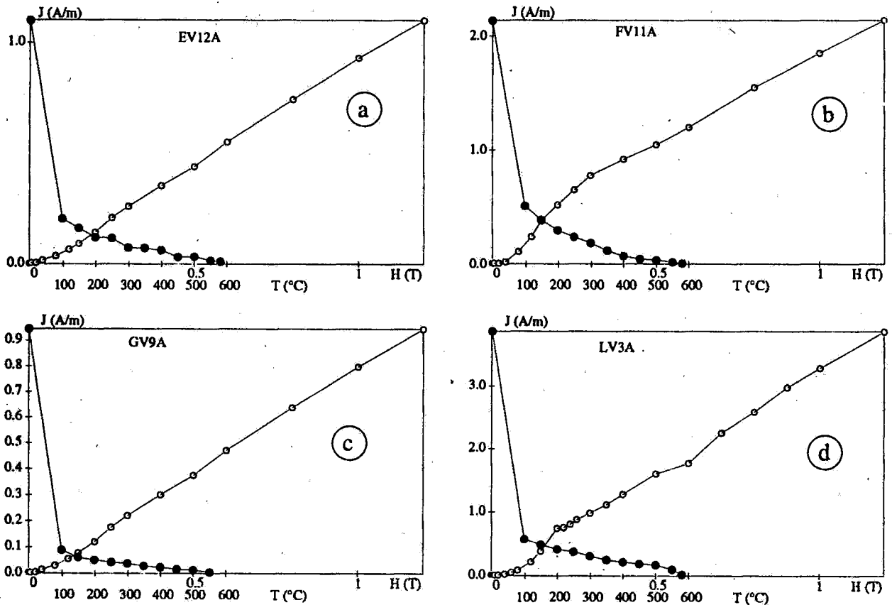
Fig. 4 - Courbes d'aimantation rémanente isotherme (ARI) à saturation (ARIs) en fonction du champ induit à 1.2 T (cercle ouvert) et leur désaimantation thermique (cercle fermé) déterminées sur des échantillons des 4 sites (a-d). La présence de minéral de type goéthite est confirmée puisqu'on détruit pratiquement 80% de la rémanence avant 100° C. Dans tous les cas, la température de blocage maximum est celle d'un minéral ayant un point de Curie voisin de 580° C, probablement de la magnétite, ce qui justifie la transformation de sulfures.
