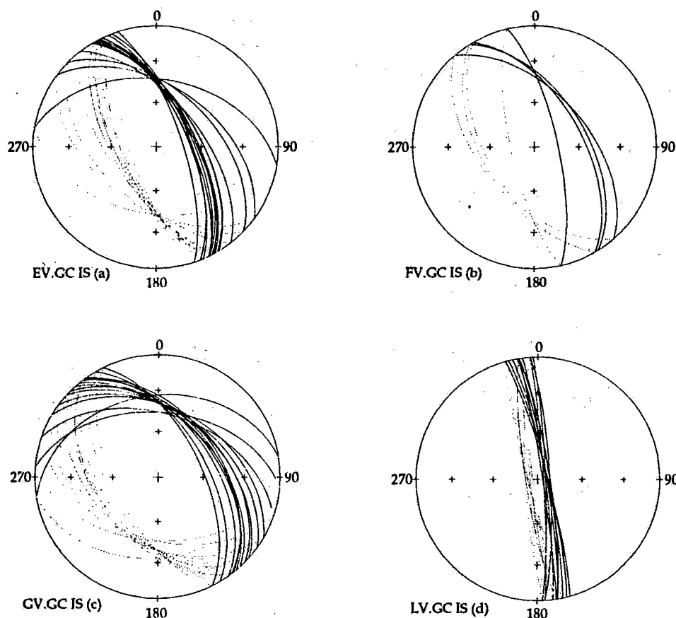
Fig. 3 - Projection à aire égale représentant les plans des grands cercles isolés par méthode de Halls (1978) sur les 4 sites (a-d) avant corrections tectoniques. La convergence de ces plans se fait lorsque l'on déplisse partiellement la structure. Les directions sont représentées dans le tableau II.
