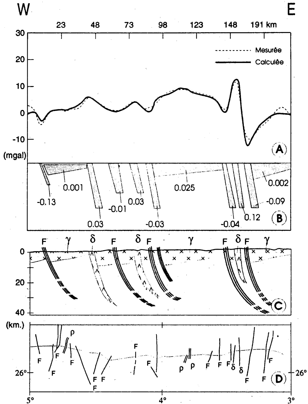
(A), (B) Modélisation des données gravimétriques. (C) Interprétation géologique possible. (D) Localisation sur le levé gravimétrique des principales failles et des principaux filons reconnus dans le socle (F: failles; p: rhyolites ou microgranites; δ: dolérites).
