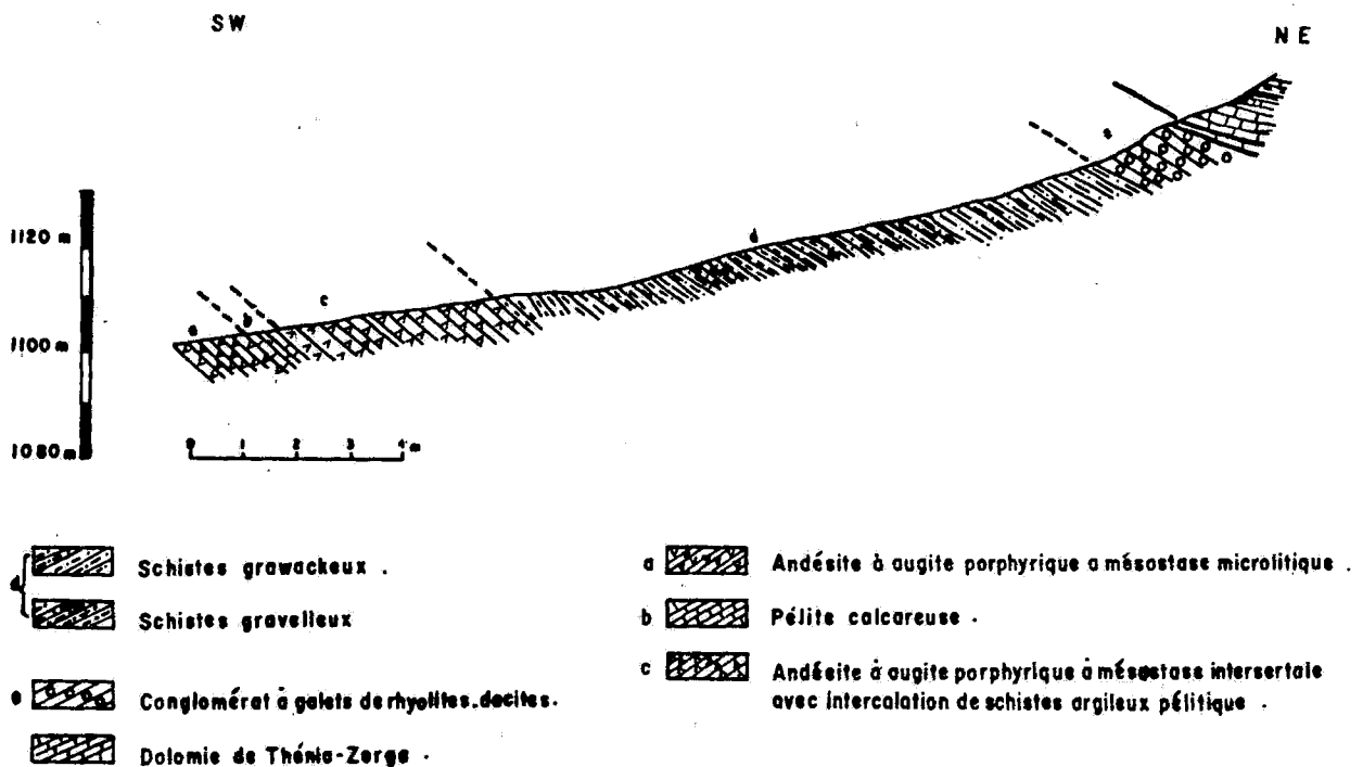
Fig. 2 - Coupe de la série de schistes de Thenia Zerga
