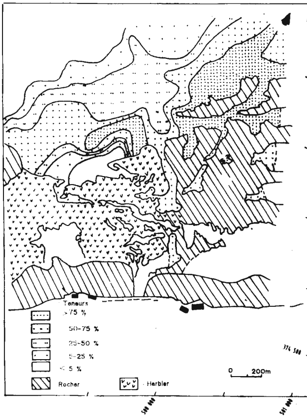
Fig. 4 - Carte de répartition du faciès bioclastique.
