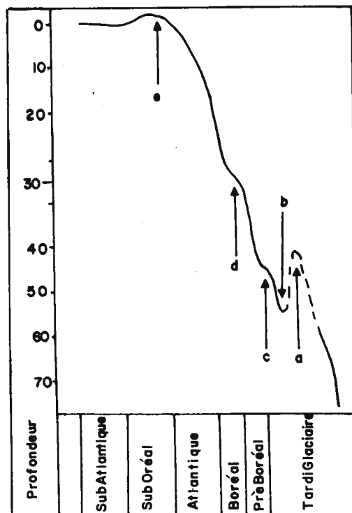
Fig. 7 - Courbe des variations du niveau marin dans le Golfe du Lion au cours de l'Holocène. (D'après ALOISI, 1986).
